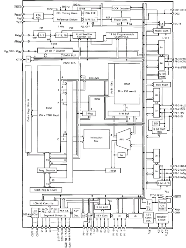
4. IC201-TC9327AF
